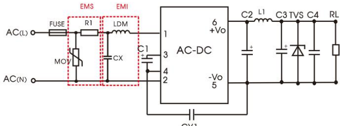
推荐电路 3
