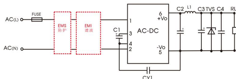
LS10 系列外围器件选型参考 (不含 EMC 器件)
