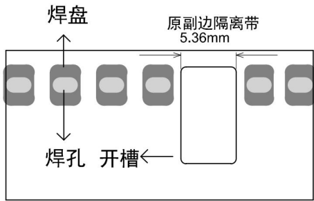
LS10-13BxxR3P 系列推荐焊盘
