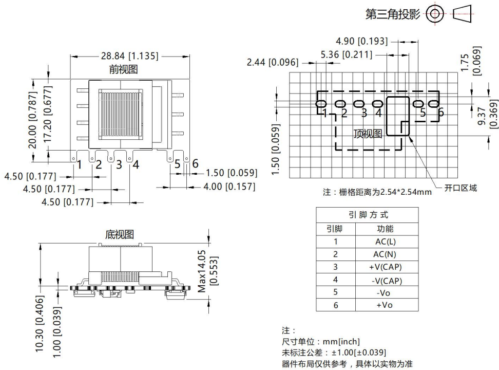
LS10-13BxxR3P 系列外观尺寸图
